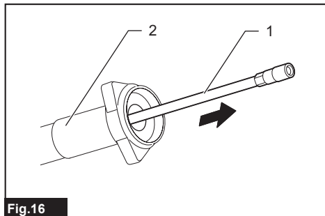
Fig.16 ► 1. Eje de núcleo flexible 2. Entubado exterior
