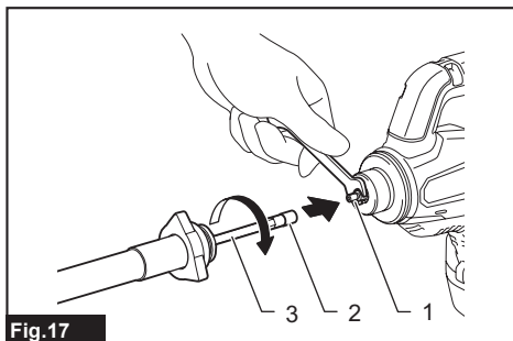
Fig.17 ► 1. Eje de transmisión 2. Acoplador de extremo 3. Eje de núcleo flexible
