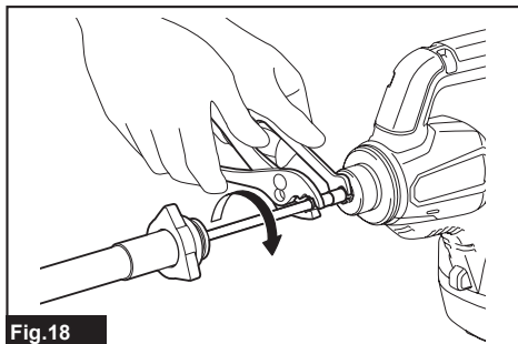
Fig.18 4. Enrosque a mano el cople del entubado exterior sobre la rosca macho de la herramienta.
